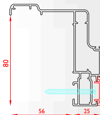
COD.GX 03 TELAIO STORICO CON CARTERINO COPRI FISSAGGIO
