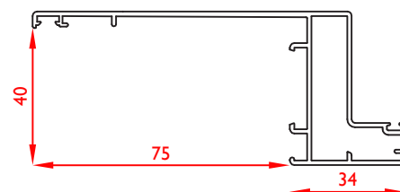
COD.TEL 75 TELAIO CON ALETTA DA mm 75
