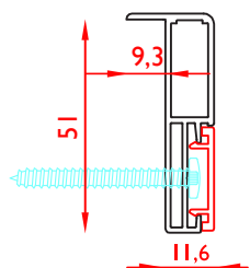
COD.TLS TELAIO A SCOMPARSA CON CARTERINO COPRI FISSAGGIO
