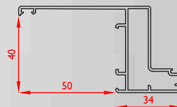
COD.TEL 50 TELAIO CON ALETTA DA mm 50
