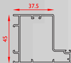
COD.TL 00 TELAIO A L MAX
