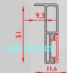
COD.TLS TELAIO A SCOMPARSA CON CARTERINO COPRI FISSAGGIO
