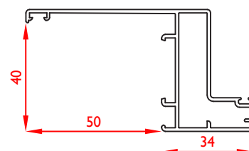
COD.TEL 50 TELAIO CON ALETTA DA mm 50
