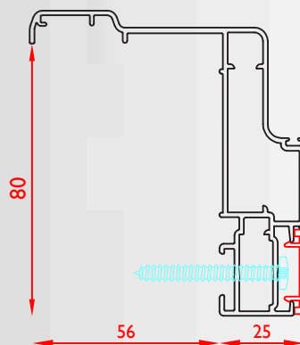
COD.GX 03 TELAIO STORICO CON CARTERINO COPRI FISSAGGIO
